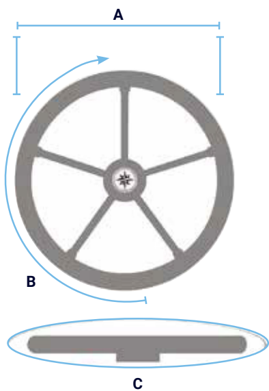
A] Diametro timone • Helm diameter B] Circonferenza totale • Helm circumference C] Ingombro totale • Total sizes
