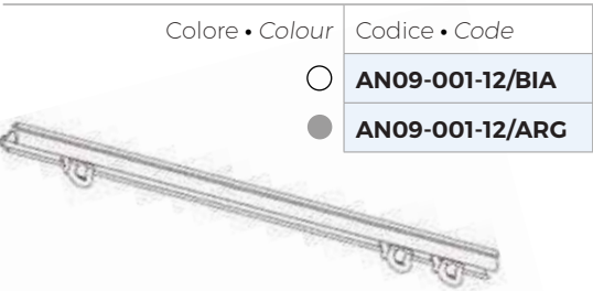
Binario in alluminio per tende leggere Profilo preforato con passo di 120 mm Colori: bianco, argento. Aluminum rail for light interior curtains Perforated profile with 120 mm pitch Colors: white, silver.
