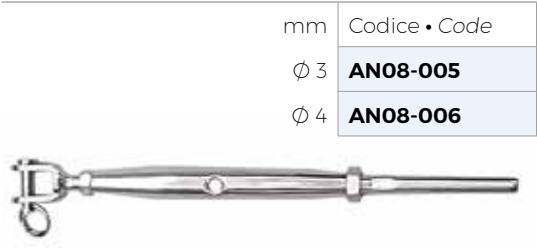
Tenditore terminale a forcella per cavo Ø 3 | 4 mm in acciaio inox AISI 316. Filettatura interna M6 Turnbuckle fork-terminal for wire cable Ø 3 | 4mm AISI 316 stainless steel. M6 Internal thread
