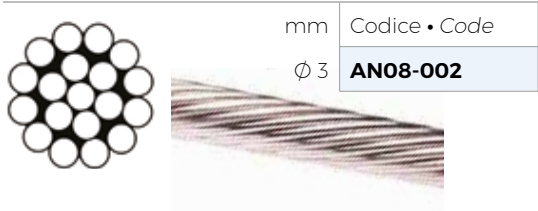
Cavo draglie in acciaio inox Ø 3mm 1x19 Stainless steel lifelines cable Ø 3mm 1x19
